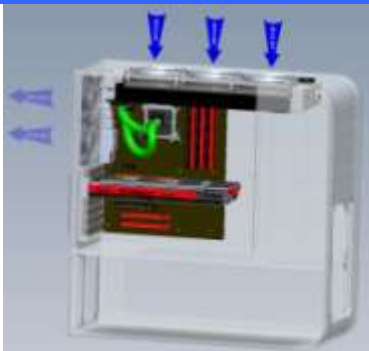
Refroidissement liquide du CPU seul
