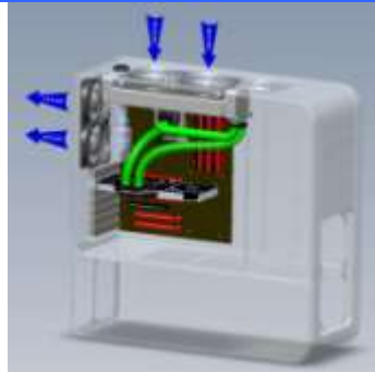
CPU + (1) Carte Graphique refroidie par eau
