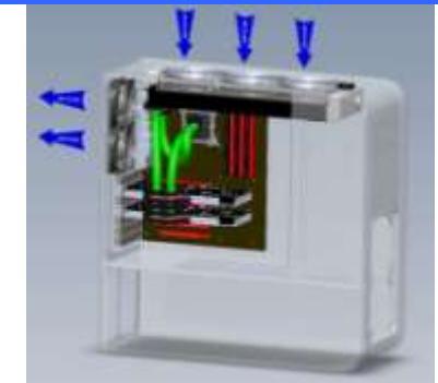
CPU + (2) Carte Graphiques refroidies par eau
